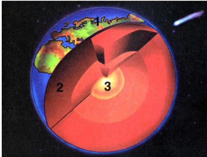
1. Litosfera: Corteza terrestre; 2. Pirofera: Zona caliente o Magna; 3. Barisfera: Núcleo central
